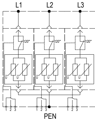
Принципиальная схема
